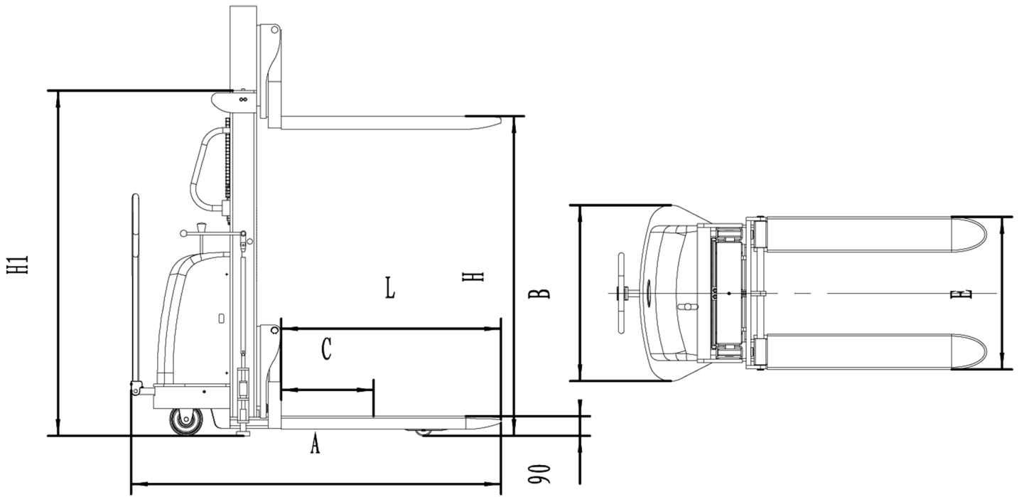
Abbildung 1. Abmessungen des Hydraulik-Staplers mit Elektroantrieb DYC.
